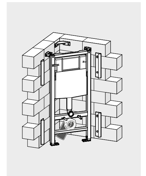
Set per il montaggio angolare
