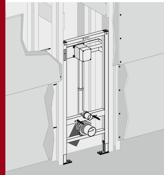
Montaggio su telaio Costruzione a secco
