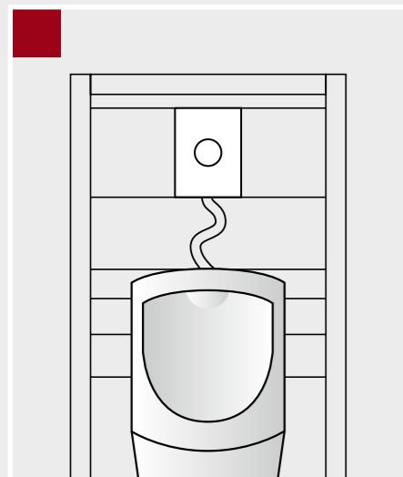
Il set per l'incasso sotto intonaco della SCHELL
