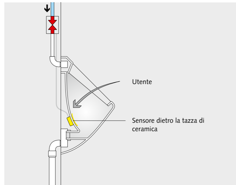
Installazione nascosta dietro la tazza in ceramica
