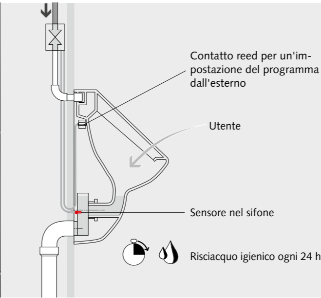
Sistema di comando elettronico per orinatoi COMPACT LC
