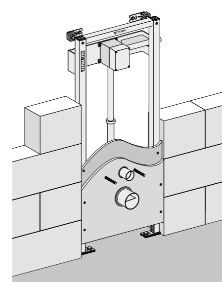
Montaggio davanti ad una parete spessa Da murare
