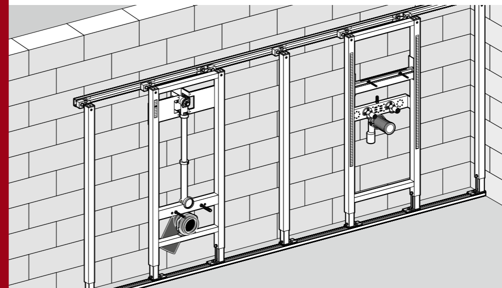
Montaggio in sistemi a traversa
