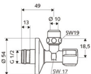
SCHELL rohový regulační ventil COMFORT Regulační ventil s dvojitou zpětnou klapkou přípoj 1/2" / DN 15
