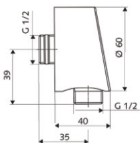
označení zboží bal. rozměr objednáací číslo povrch SCHELL nástěnné připojovací koleno PURIS Designové provedení přípoj 1/2" / DN 15, vývod 1/2" / DN 15
