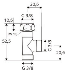
SCHELL T-kus 3/8" x 3/8" x 3/8" / DN 10 s jednou převlečnou maticí 3/8"
